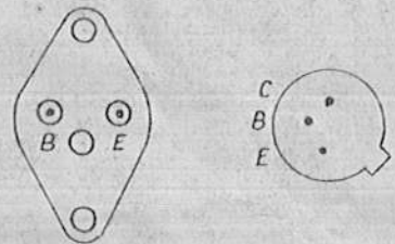
Sockelschaltbilder
