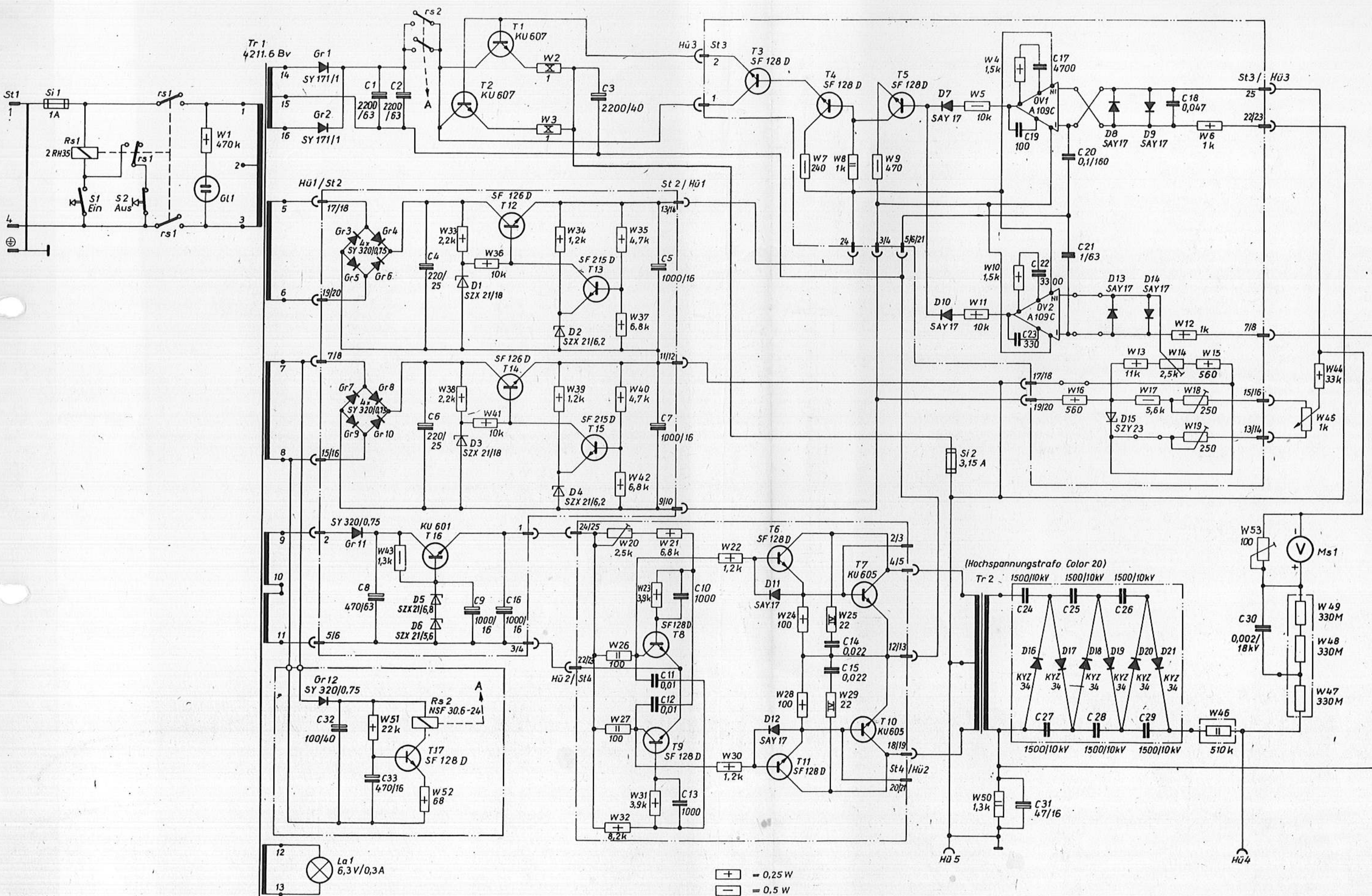
Gleichspannungsregler Typ 4211 +25 kV max. 1mA
