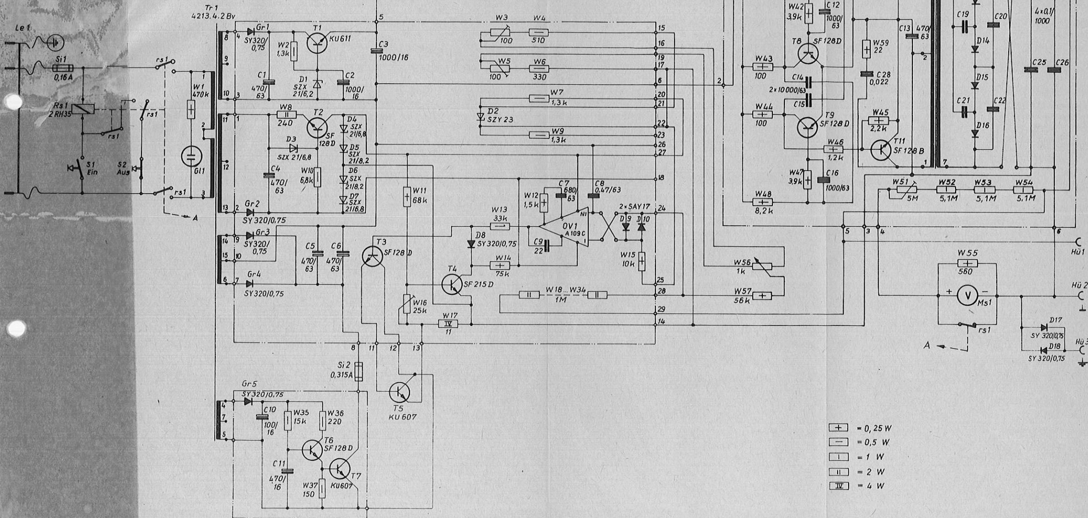
Gleichspannungsregler Typ 4214
